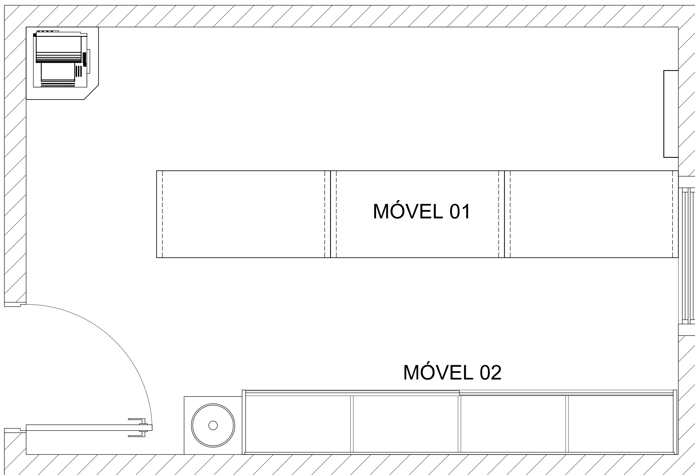
PLANTA BAIXA SALA ESCALA .....1:15
